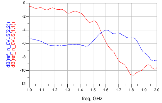
REF-IN-0V Decoupling
