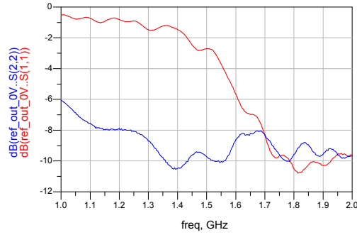
REF-OUT-0V Isolation
