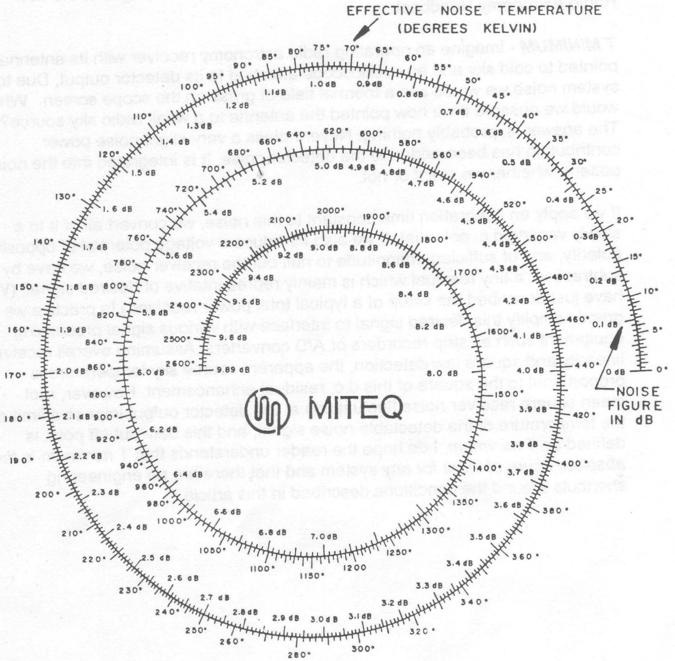
Umrechnung Rauschmaß [dB] - Rauschtemperatur [K]
